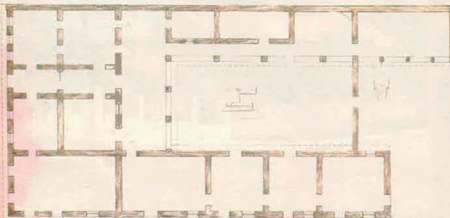
Planta Baixa da Casa de Amarante.
